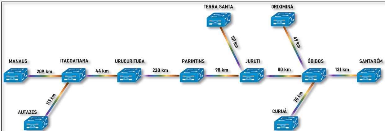
Figura 3. Diagrama de rede óptica de longa distância da Infovia 01.
